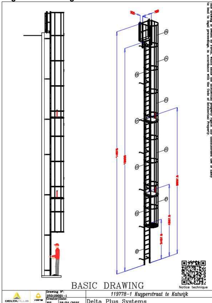
Figuur 2: Tekening koilladder.
